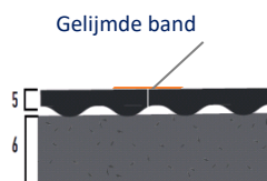
4. Alternatief detail voeg (tegen elkaar)
