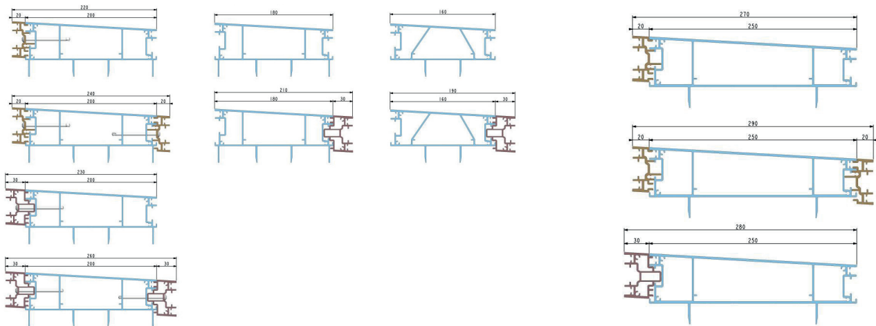
Principe d'extensions sur profils Omega 3 en 160, 180 et 200
