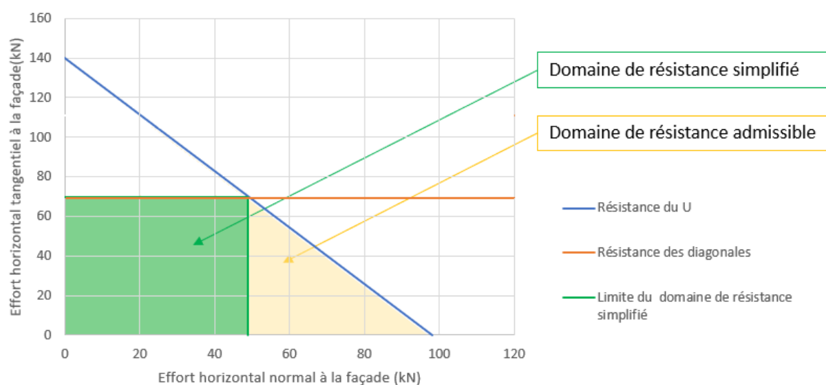
Figure 16 Domaine de résistance admissible du modèle HI / HIP / HIB 1.12/2X2.8
