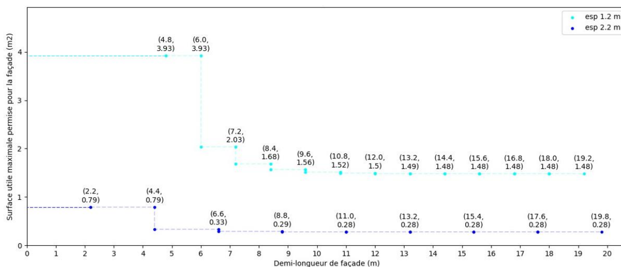
Figure 22 Domaines admissibles vis-à-vis de la sollicitation thermomécanique pour les rupteurs parasismiques avec diagonales \varnothing = 12 mm (HI/HIP/HIB 1.12/2x2.12)
