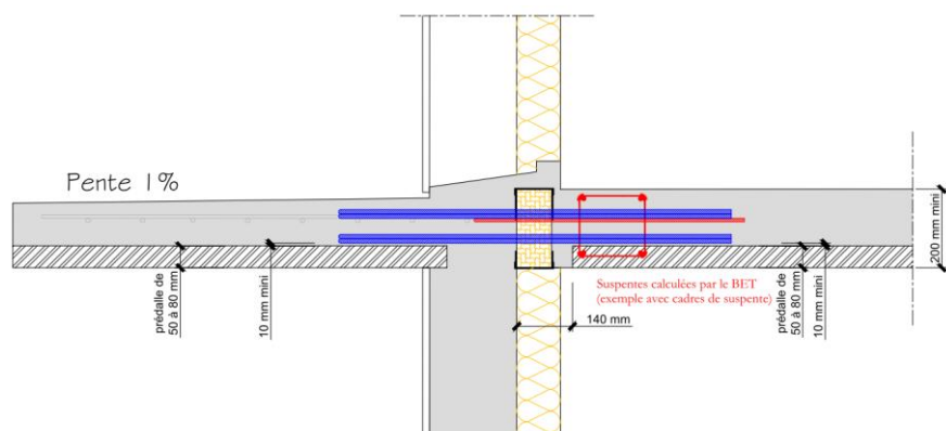
Figure 14 : Coupe de principe d'application HIB avec prédalles BA ou précontraintes de chaque côté
