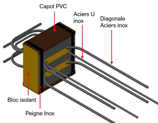
Figure 1 : Rupteur ISOTEC RT+ sismique - modèle HI (Voir Annexe 1)
