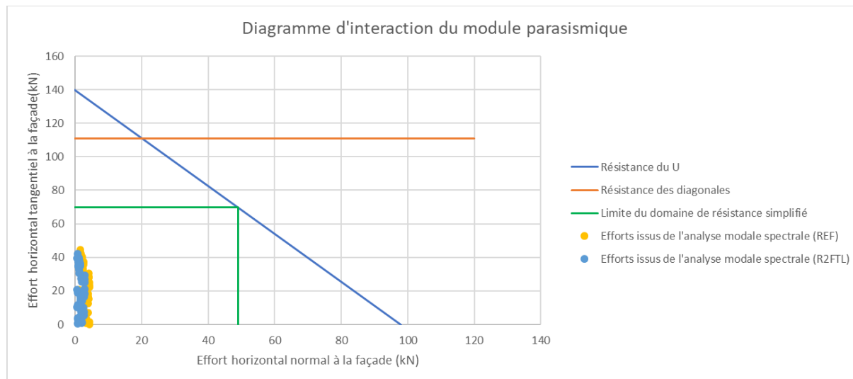
Figure 30 Vérification de la résistance des rupteurs parasismiques vis à vis du séisme
