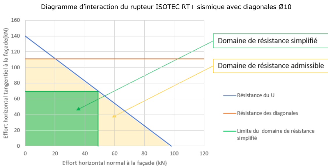
Figure 17 Domaine de résistance admissible du modèle HI / HIP / HIB 1.12/2X2.10
