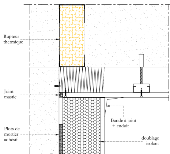
Figure 34 : Mise en œuvre d'isolation périphérique sur des ouvrages de plâtrerie
