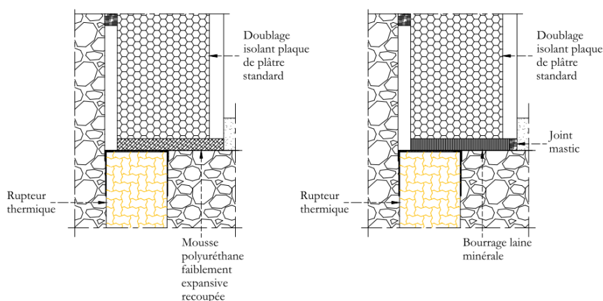
Mise en œuvre d'isolation périphérique sur des ouvrages de plâtrerie
