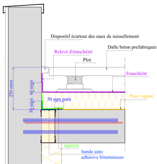
Figure 31 : Coupe sur pare-vapeur ou revêtement d'étanchéité bitumineux soudé à la flamme (élément dalle-façade)
