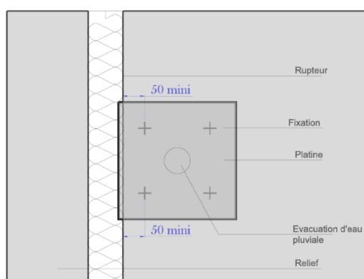
Figure 32 : Réserve avec rupteur continu posé en plancher
