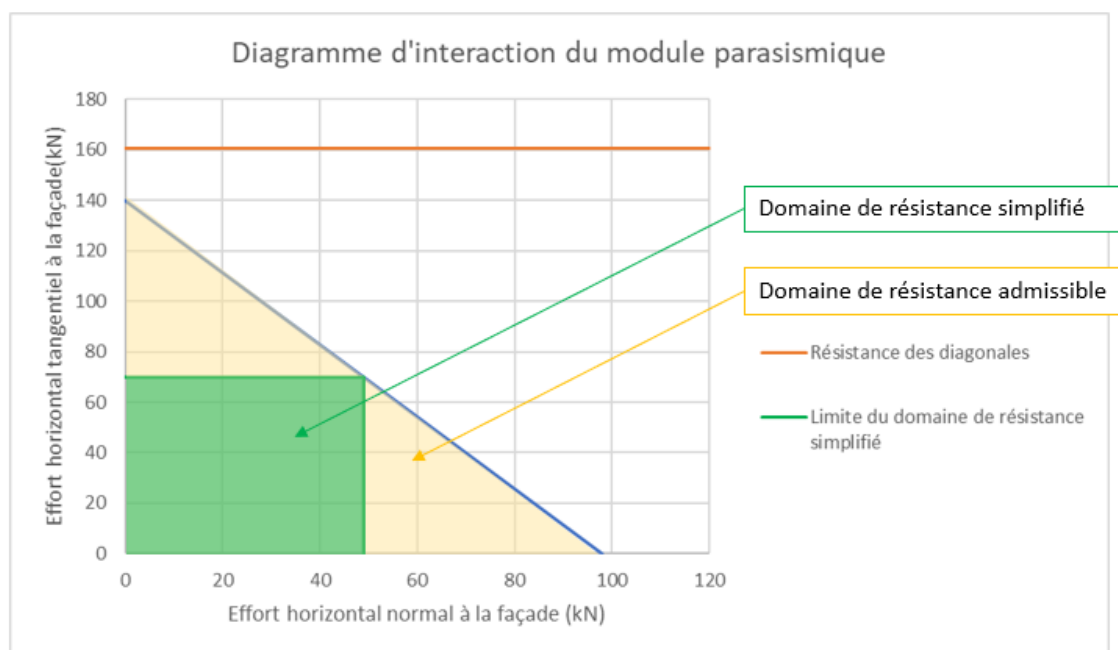
Figure 18 Domaine de résistance admissible du modèle HI / HIP / HIB 1.12/2X2.12
