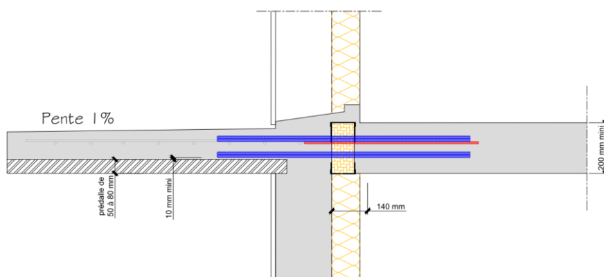
Figure 13 : Coupe de principe d'application HIB avec prédalle BA ou précontrainte côté balcon
