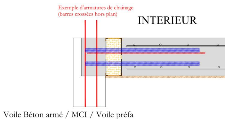
Figure 8 : Coupe type du rupteur « ISOTEC RT+ Sismique » - liaison dalle coulée en place-façade (HI)
