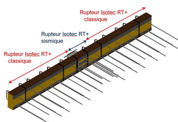
Liaison façade - plancher
