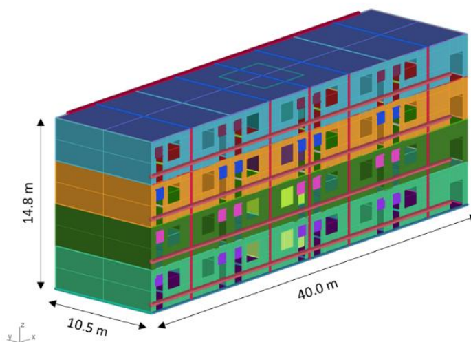
Figure 24 : Vue en perspective du modèle et dimensions principales
