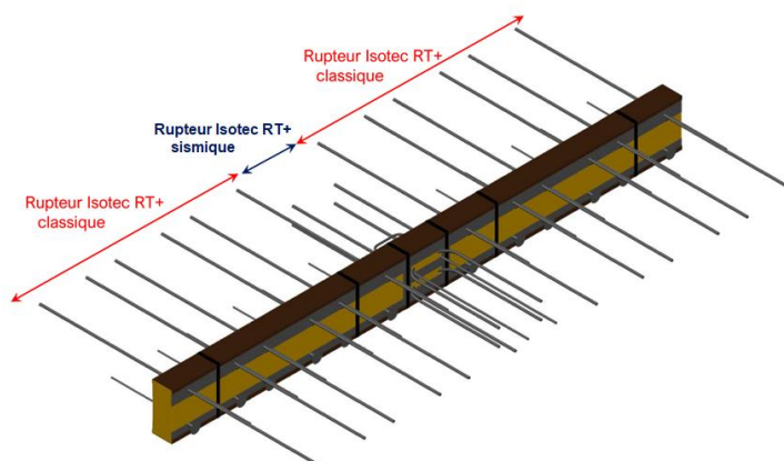
Liaison balcon - plancher
