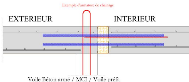
Figure 4 : Coupe type du rupteur ISOTEC RT+ sismique - liaison dalle-balcon (HIB)
