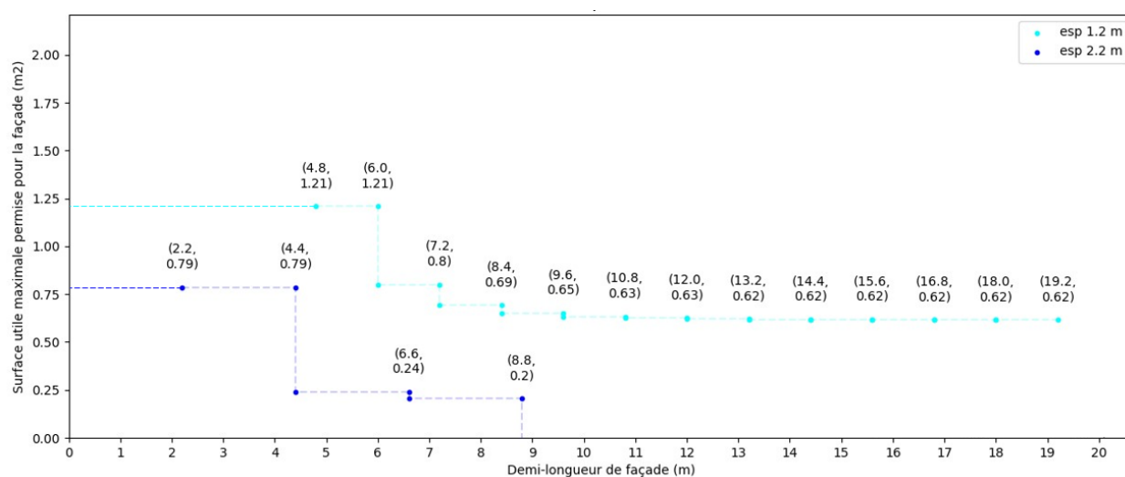
Figure 21 Domaines admissibles vis-à-vis de la sollicitation thermomécanique pour les rupteurs parasismiques avec diagonales \varnothing = 10 mm (HI/HIP/HIB 1.12/2x2.10)
