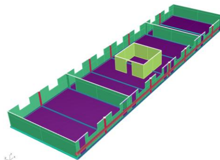
Figure 25 : Coupe en perspective du modèle
