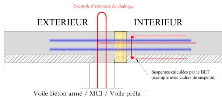
Figure 6 : Coupe type du rupteur « ISOTEC RT+ Sismique » - liaison prédalle balcon (HIB)
