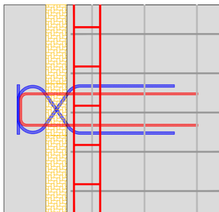
Figure 10 : Coupe de principe du Rupteur ISOTEC RT+ sismique - modèle HIP assorti des cotes dimensionnelles
