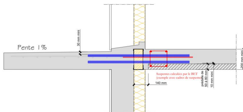
Figure 12 : Coupe de principe d'application HIB avec prédalle BA ou précontrainte côté dalle intérieure
