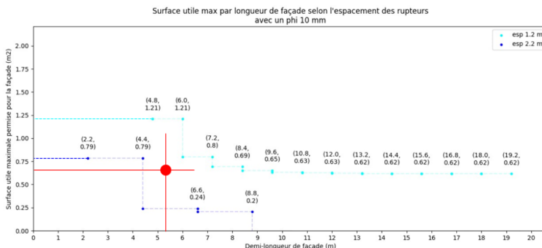
Figure 29 Dimensionnement du bridage thermomécanique par rupteurs « ISOTEC RT+ Sismique » dans les murs pignons du bâtiment exemple
