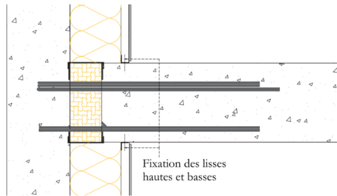
Figure 35 : Disposition avec doublage à ossature métallique
