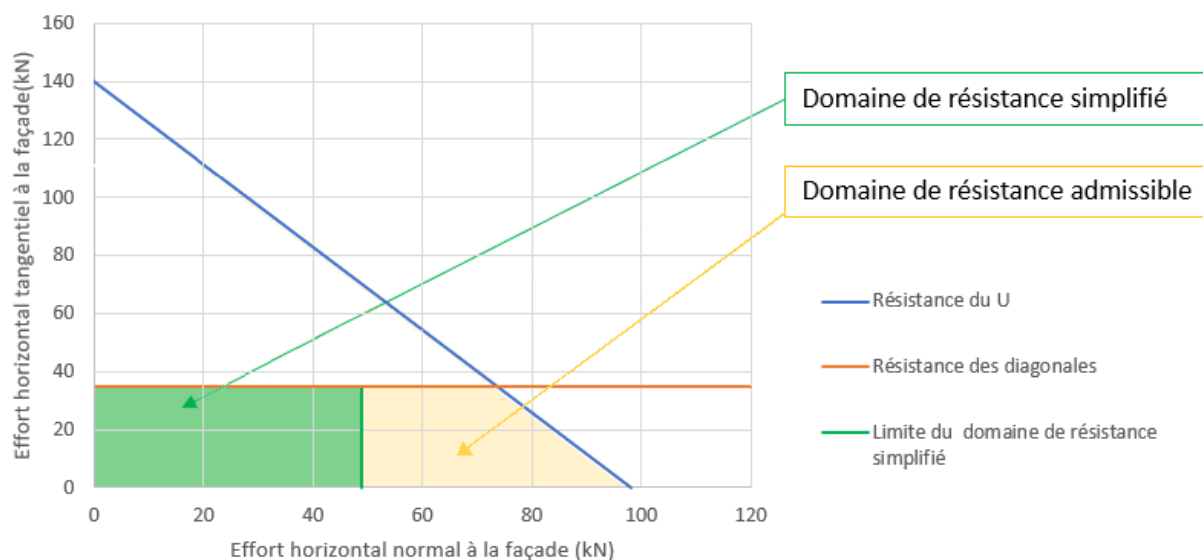
Diagramme d'interaction du rupteur « ISOTEC RT+ Sismique » avec diagonales Ø6
