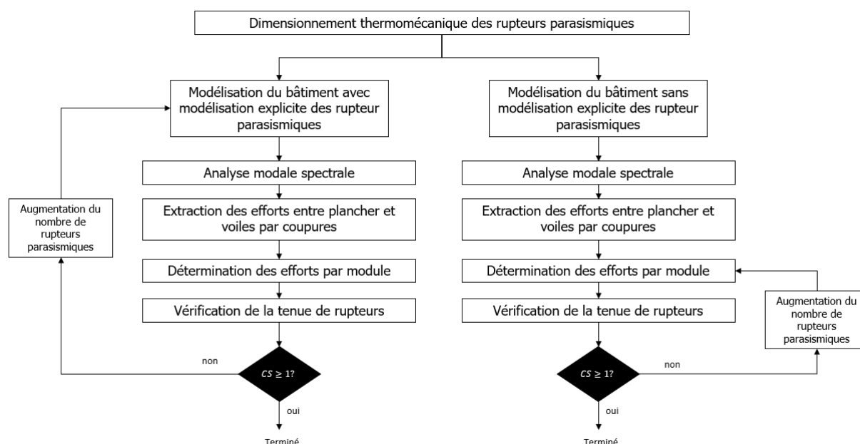
Figure 23 Organigramme de dimensionnement des rupteurs ISOTEC RT+ sismiques
