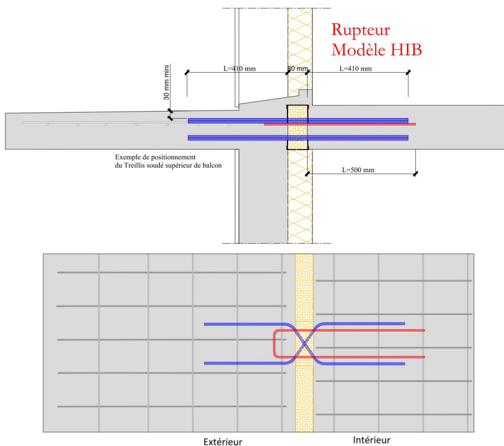
Figure 11 : Coupe de principe du Module HIB assorti des cotes dimensionnelles
