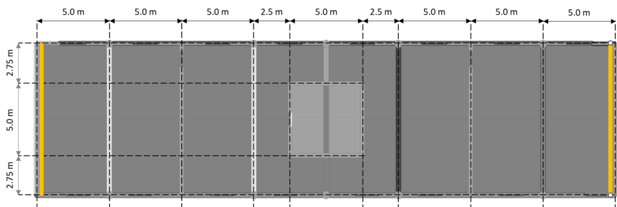
Figure 28 Murs de pignon ( L = 10.5 m) pour le dimensionnement d'un bridage thermomécanique par rupteurs ISOTEC RT+ sismiques
