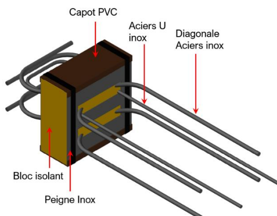
Figure 2 Rupteur « ISOTEC RT+ Sismique » - modèle HIP (Voir Annexe 2).
