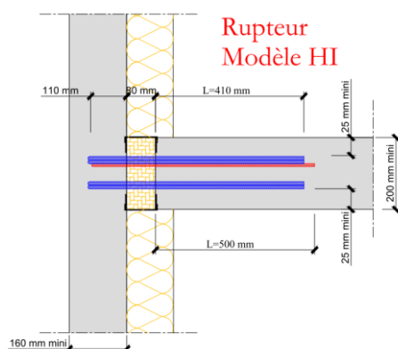
Figure 9 : Coupe de principe du Rupteur « ISOTEC RT+ Sismique » - modèle HI assorti des cotes dimensionnelles
