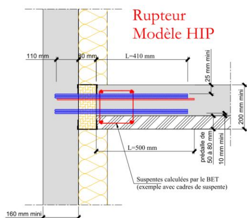
Figure 10 : Coupe de principe du Rupteur ISOTEC RT+ sismique - modèle HIP assorti des cotes dimensionnelles
