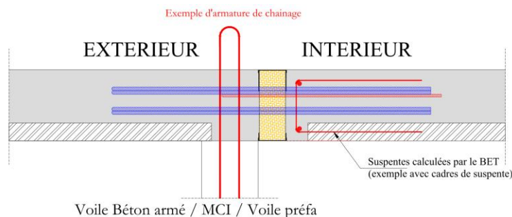
Figure 5 : Coupe type du rupteur « ISOTEC RT+ Sismique » - liaison prédalle décalée balcon (HIB)
