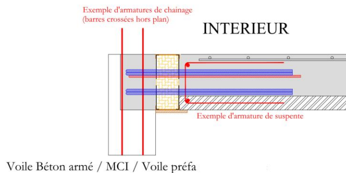
Figure 7 : Coupe type du rupteur « ISOTEC RT+ Sismique » - liaison prédalle-façade (HIP)
