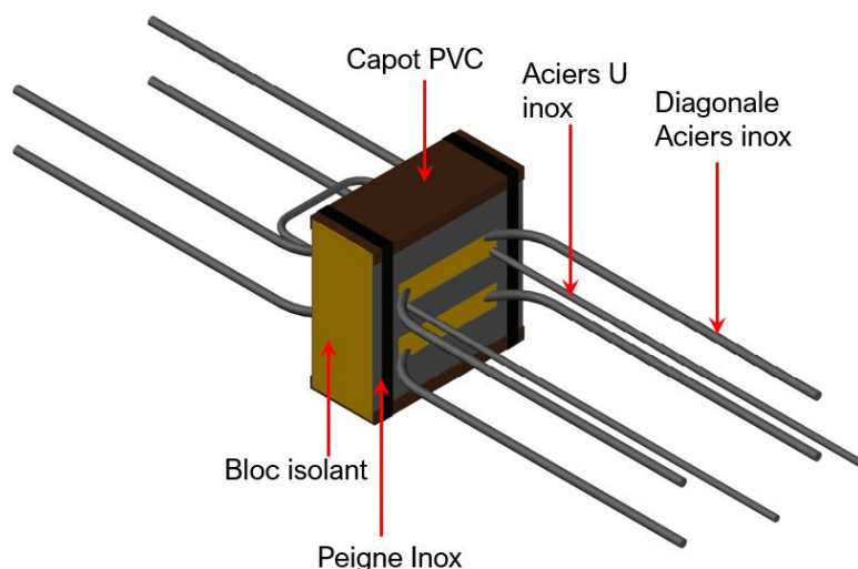
Figure 3 Rupteur « ISOTEC RT+ Sismique » - modèle HIB (Voir Annexe 3)
