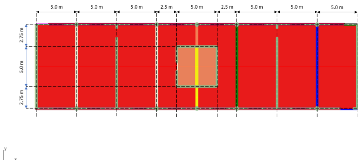
Figure 27 Dimensions de l'ouvrage
