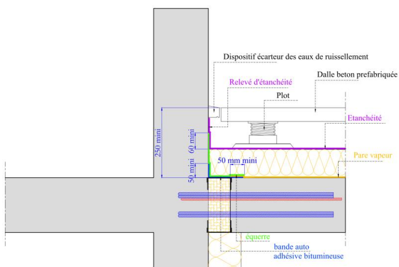
Figure 33 : coupe sur pare-vapeur ou revêtement d'étanchéité bitumineux soudé à la flamme (élément dalle-balcon)
