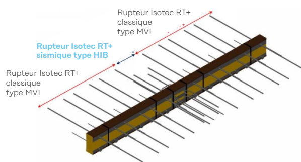
Liaison dalle-balcon : combinaison rupteurs classiques MVI + rupteurs sismiques HIB
