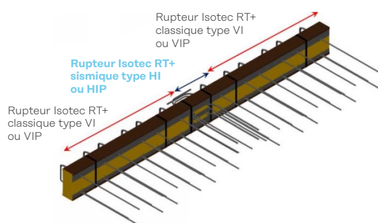
Liaison dalle-façade : combinaison rupteurs classiques VI(P) + rupteurs sismiques HI(P)
